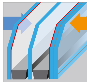
Verbundsicherheitsglas VSG 6 mm einseitig außen mit 3-fach Wärmeschutzverglasung , Ug 0.7 W/mK
